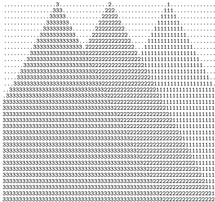
FIGURE 3 – L'automate « max » (ou encore, l'automate des « pots de peinture renversés »). Il s'agit d'un automate sur l'ensemble \mathbb{Z} , la valeur vide est 0 et la fonction d'évolution est f(a, b, c) = \max\{a, b, c\} . Les valeurs vides sont représentées par des « . ».
