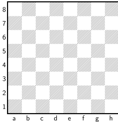
(a) L'échiquier concret dans lequel chaque case est désignée par un couple.
