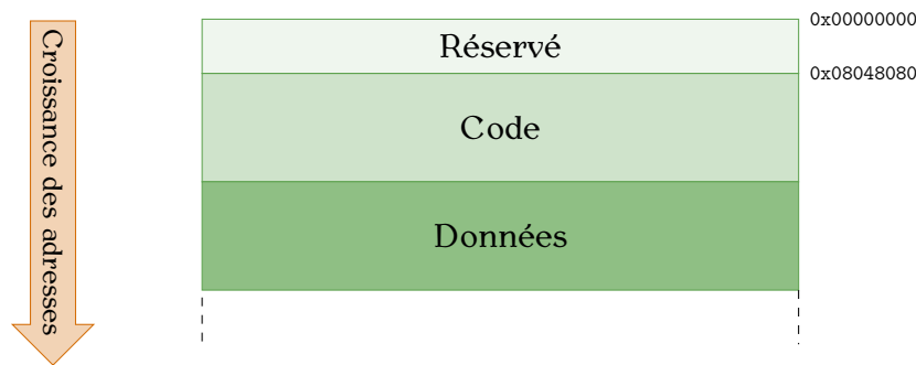
FIGURE 5 – Mémoire occupée par le programme lors de son exécution.
